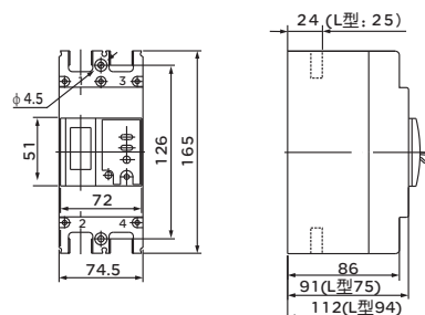
图8b RDM1L-250M/2300
